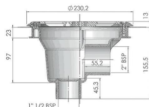
Réf. 42312 Vue de profil
