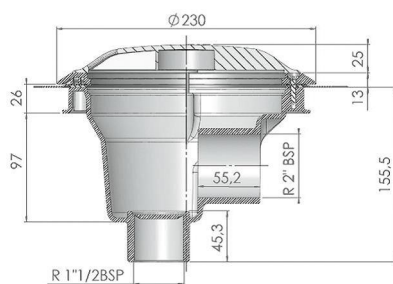
Réf. 42314 Vue de profil
