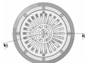
Réf. 42312 Vue de dessus
